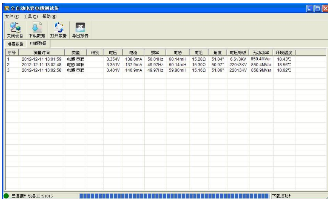
图 4.10 电感测试数据
