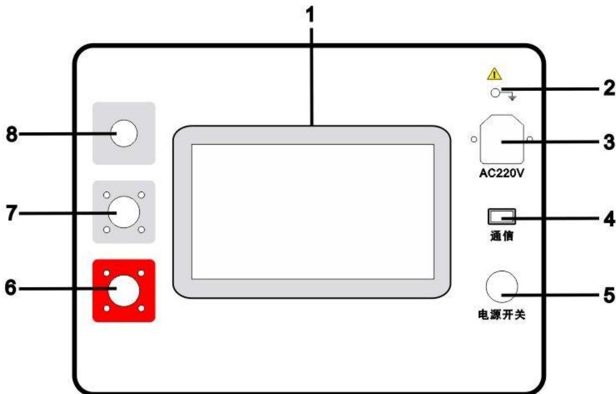
图 1.1 面板结构图
