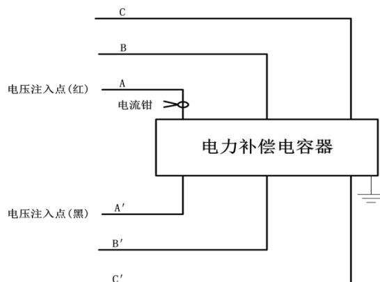
图 2.10 III型连接被试电容A 相测量接线
