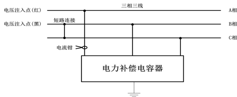
图 2.4 △形连接被试电容 A 相测量接线
