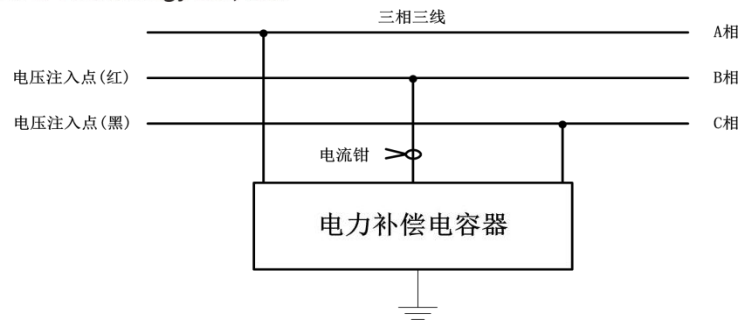
图 2.2 Y 形连接被试电容B 相测量接线
